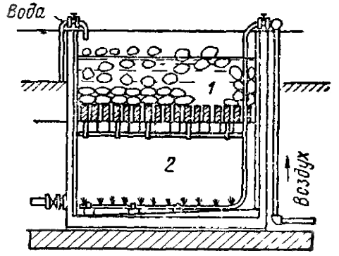
Поперечный разрез
