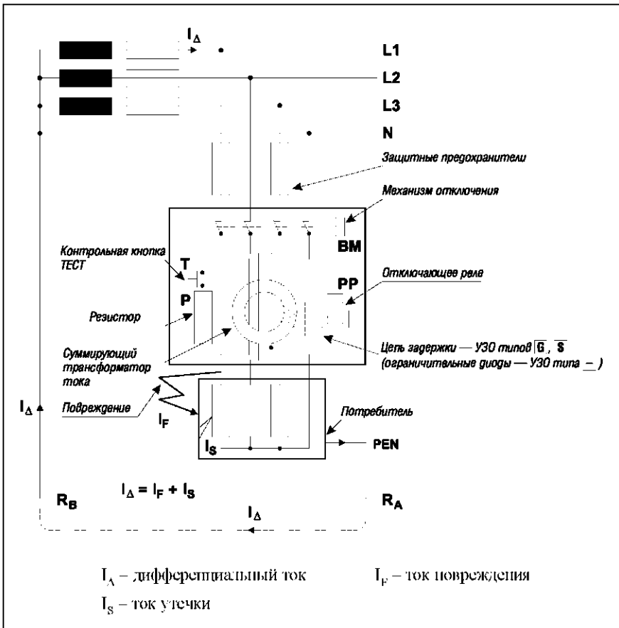
Рис. 10 Принципиальная схема подключения УЗО (сеть системы TT)
