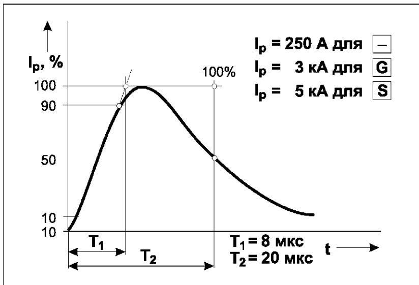
Рис. 40 Нормализованная форма ударной волны тока 8/20 мкс 1)
