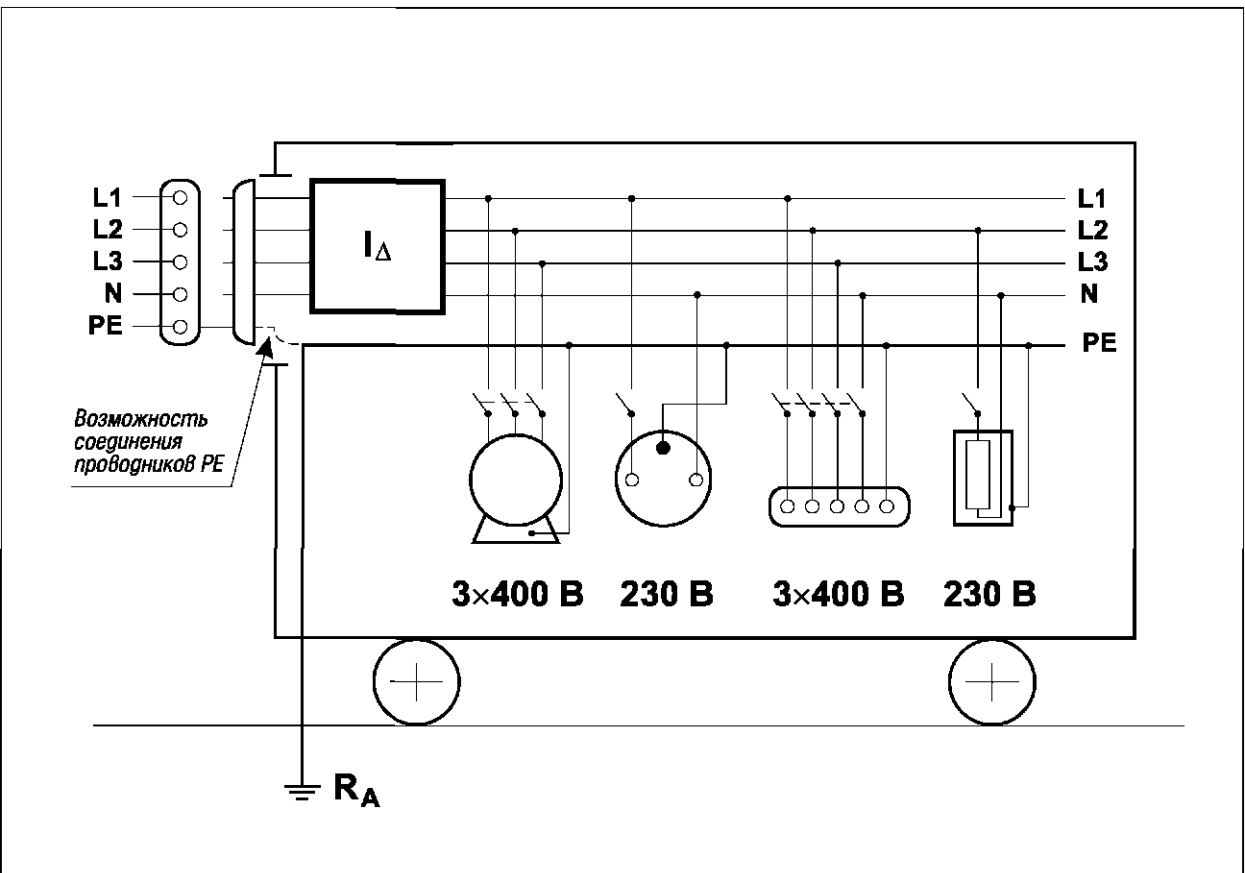
Рис. 44 Мобильные подстанции с питанием от наружного источника
