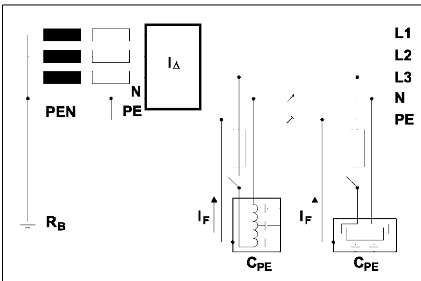
Рис. 41 Возникновение токов утечки через емкость СРЕ при коммутациях
