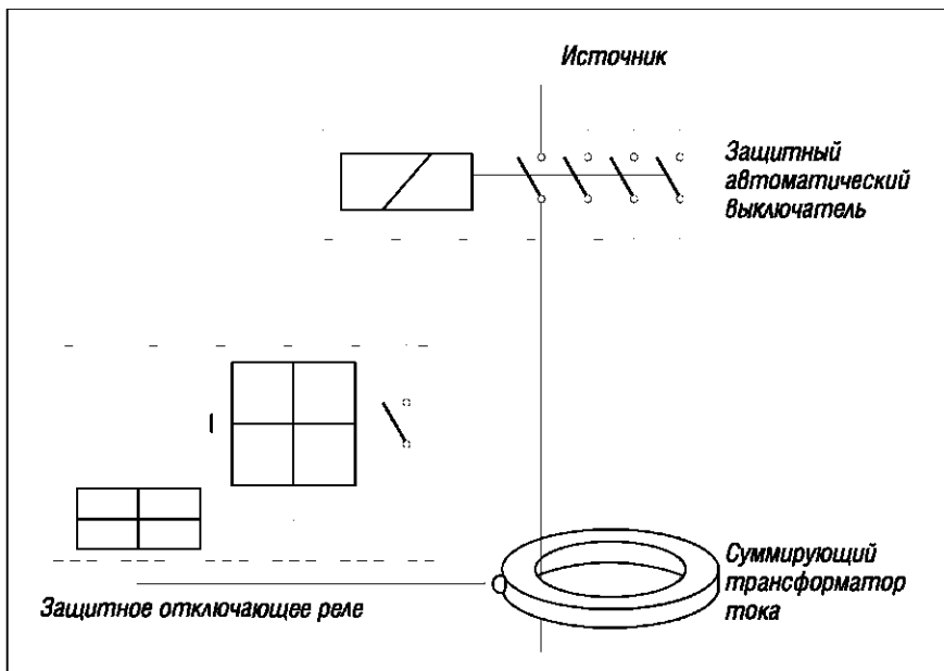
Рис. 13 Структурная схема УЗО с прямым отключением.
