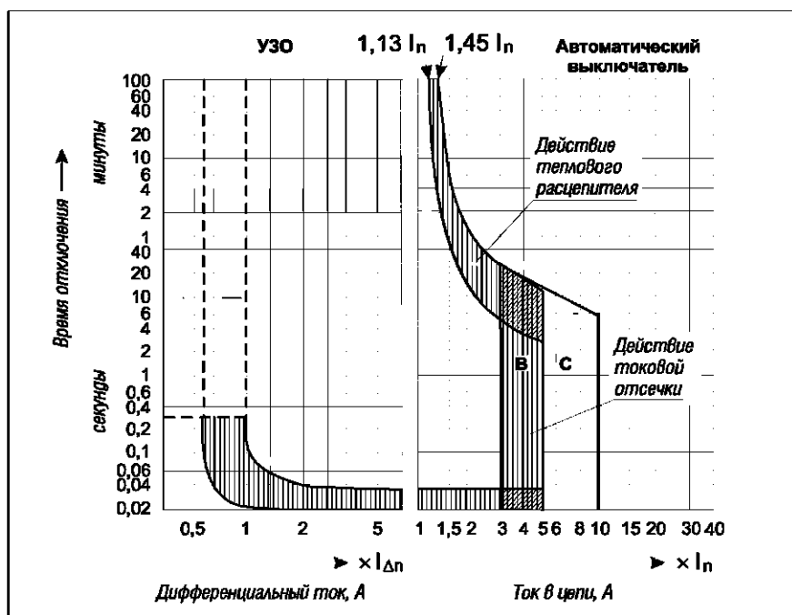
Рис. 22 Время-токовые характеристики УЗО ( I_{\Delta n} = 30 \text{ мА} ) со встроенным автоматическим выключателем.
