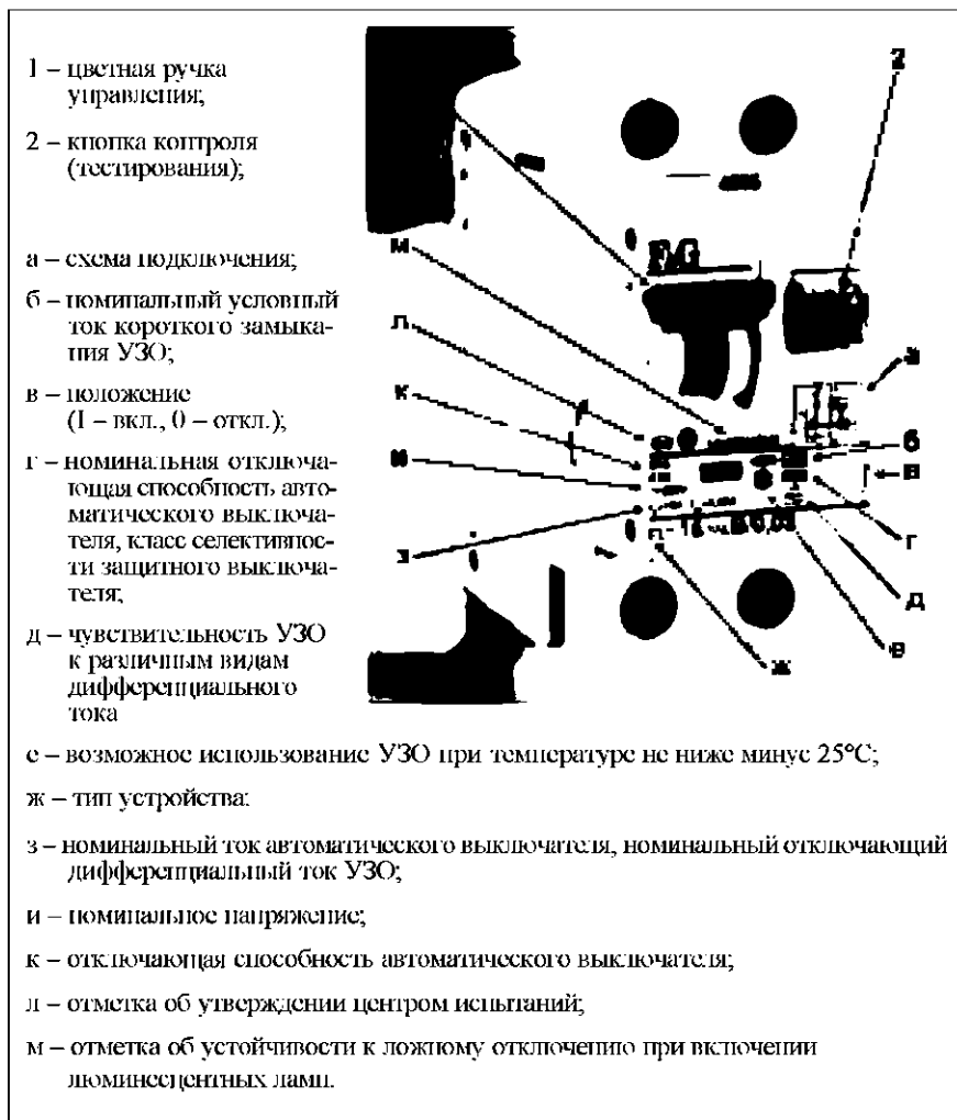
Рис. 23 Отметки на корпусе УЗО со встроенной максимальной токовой защитой
