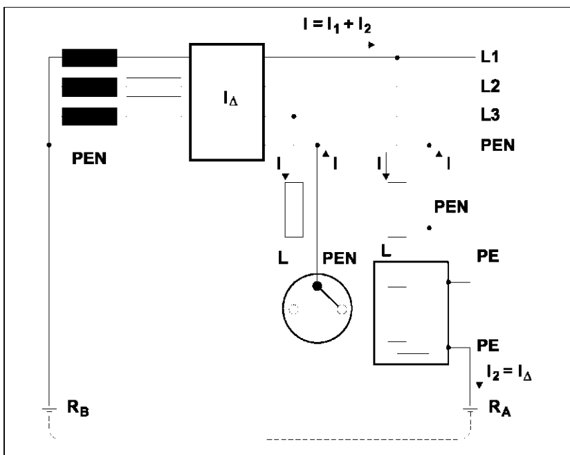
Рис. 39 Недопустимые подключения УЗО в сети TN-C
