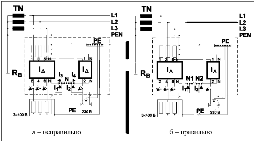
Рис. 38 Параллельное соединение УЗО
