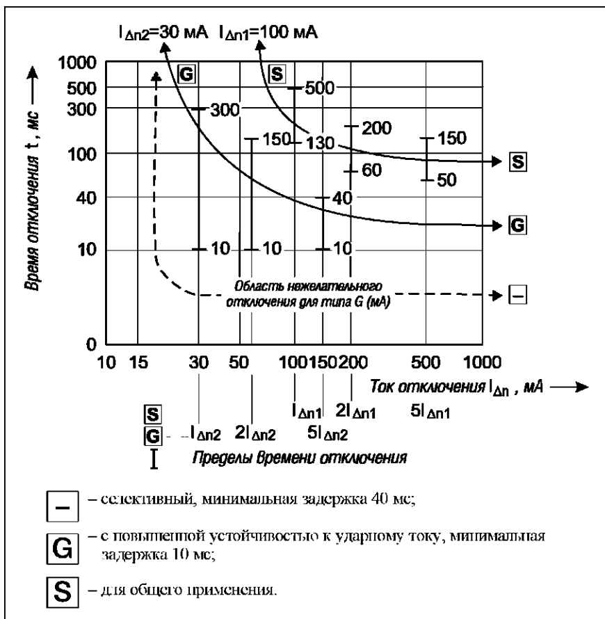
Рис. 19 Время-токовые характеристики УЗО типов G, S и общего применения
