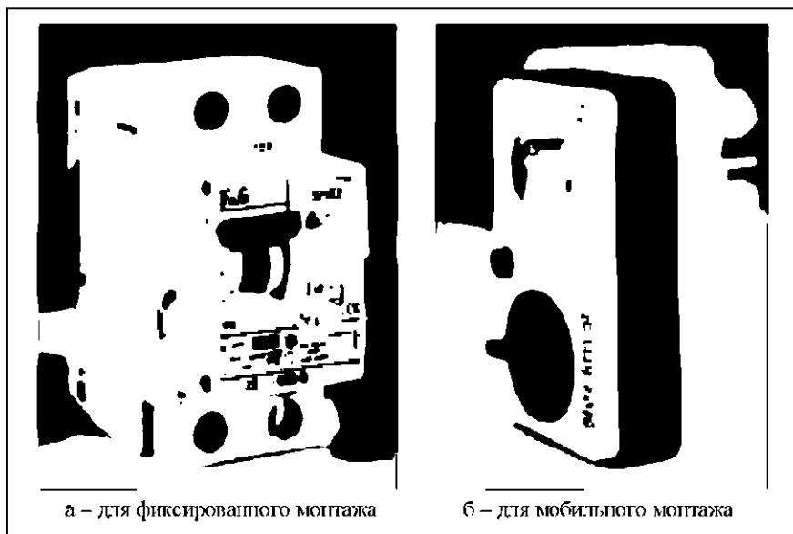
Рис. 12 Внешний вид УЗО для фиксированного и мобильного монтажа
