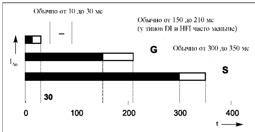
Рис. 31 Обычно значения времени отключения УЗО при испытании дифференциальным током, равным I_{\Delta n}
