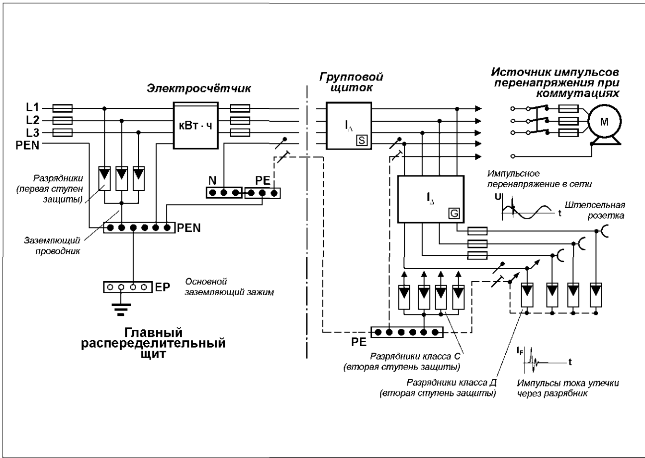
Рис. 42 Возникновение ложных отключений УЗО в электропроводке с устройствами защиты от перенапряжений.
