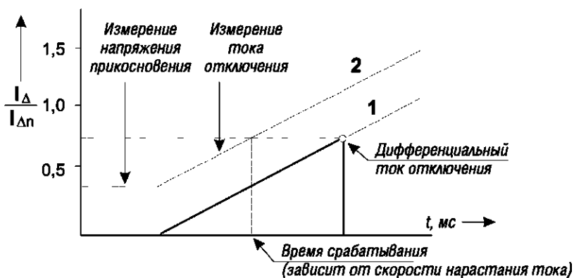
Рис. 30 Зависимости нарастания значения тока от времени при определении минимального отключающего дифференциального тока УЗО
